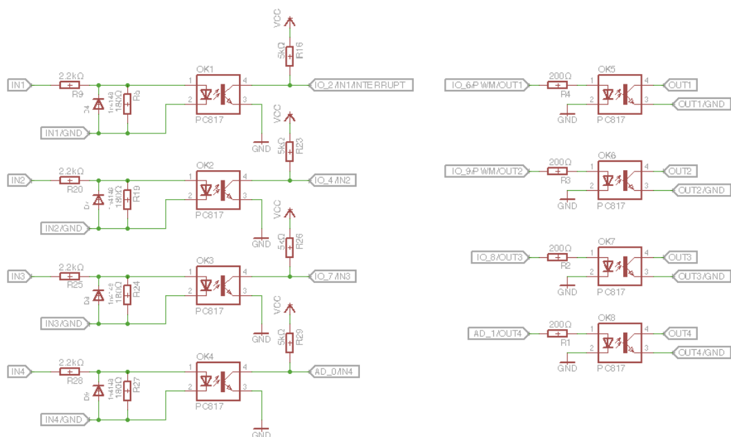
Schema, optiska in- och utgångar
