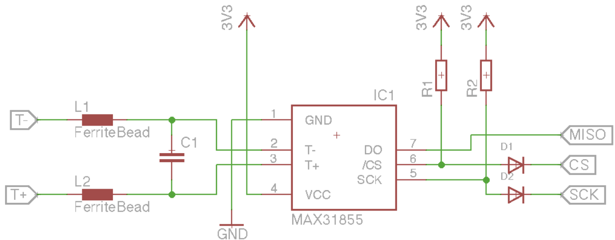
Figur 3, schematisk vy
